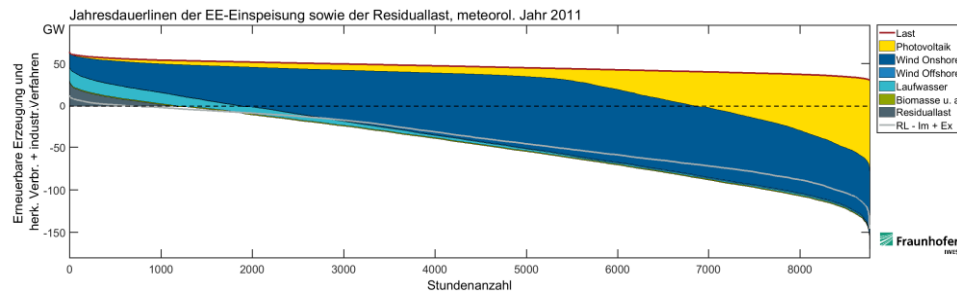
Abbildung 4-15: Jahresdauerlinie EE und unflexibler Verbrauch Wetterjahr 2011 in Frankreich, Szenariojahr 2050
