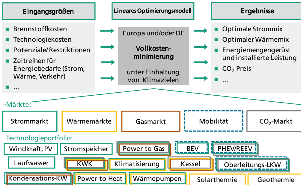
Abbildung 2-1: Schematische Darstellung der sektoriübergreifenden Ausbauplanung SCOPE
