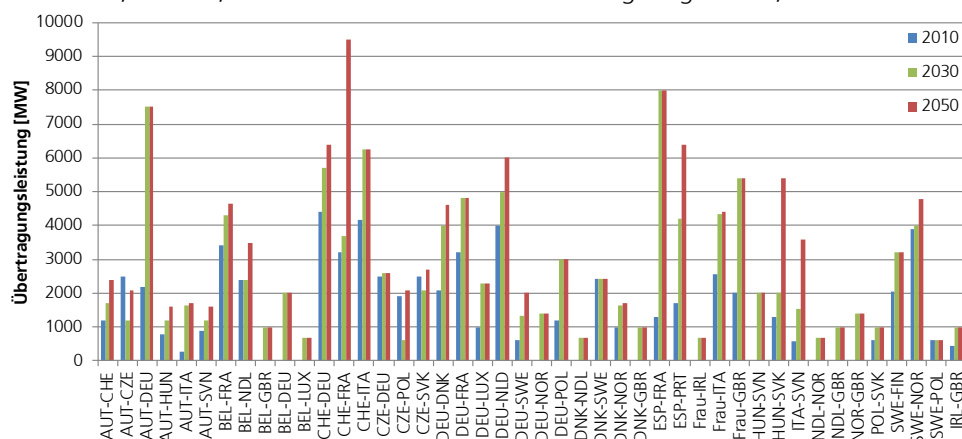
Abbildung 3-6: Kuppelleistungskapazitäten NTC in Europa
