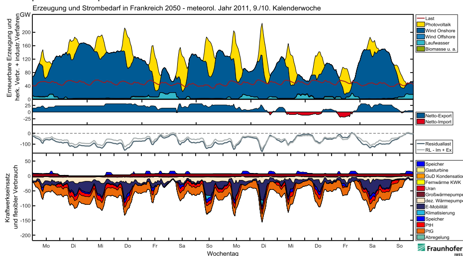
Abbildung 4-13: Verbrauch und Lastdeckung – zwei Beispielwochen Wetterjahr 2011 in Frankreich, Szenariojahr 2050
