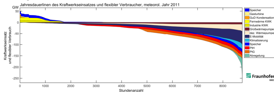
Abbildung 4-16: Jahresdauerlinie flexible Kraftwerke und flexibler Verbrauch Wetterjahr 2011 in Deutschland, Szenariojahr 2050
