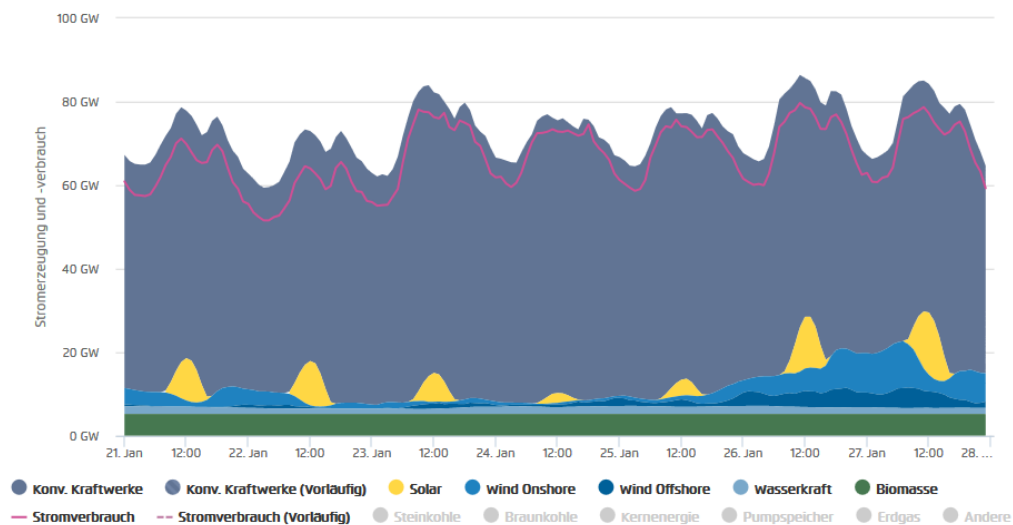
Abbildung 1-1: Beispielhafte Dunkelflaute im Januar 2017 (1 Woche So-Fr.)
