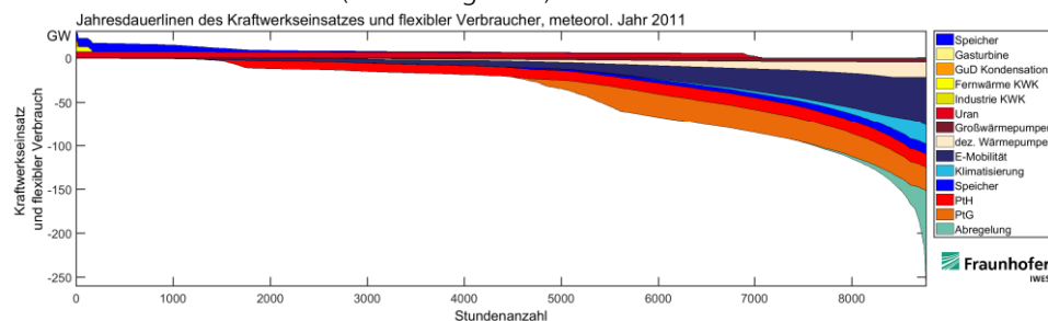
Abbildung 4-17: Jahresdauerlinie flexible Kraftwerke und flexibler Verbrauch Wetterjahr 2011 in Frankreich, Szenariojahr 2050
