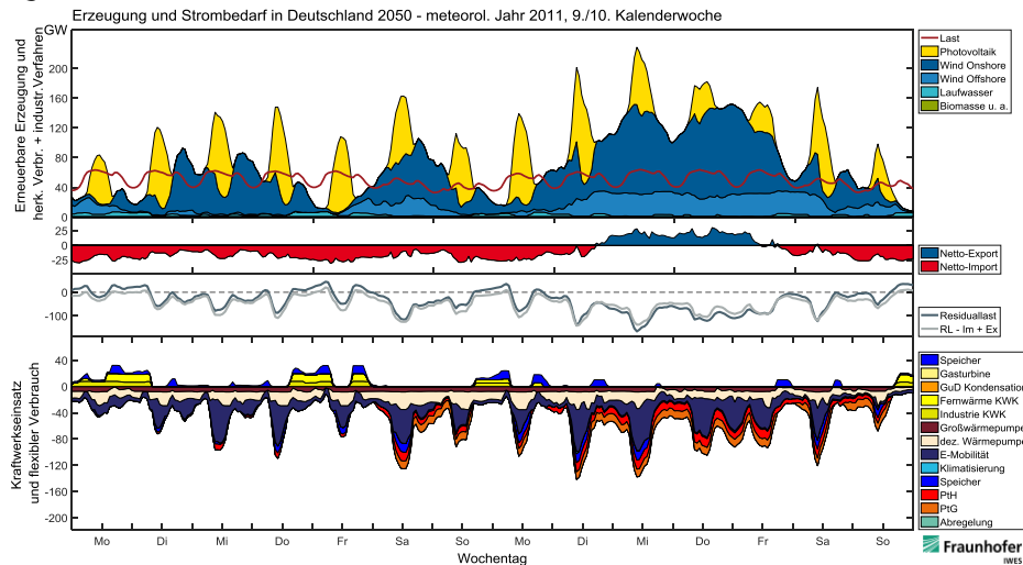
Abbildung 4-12: Verbrauch und Lastdeckung – zwei Beispielwochen Wetterjahr 2011 in Deutschland, Szenariojahr 2050 – Fokus Import/Export
