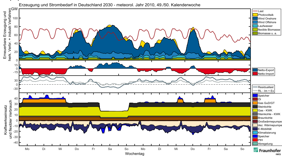
Abbildung 4-38: Zeitpunkt mit dem höchstem Kraftwerksabruf im Szenariojahr 2030, am Di. 07.12. – europäische Versorgungssicherheit
