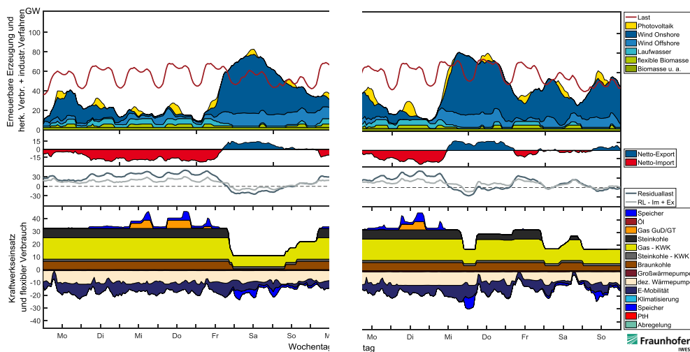
Abbildung 4-37: Zeitpunkt mit einem sehr hohen Kraftwerksabruf im Szenariojahr 2030, am Do. 07.01. (links) und Di. 26.01.2010 (rechts) – europäische Versorgungssicherheit
