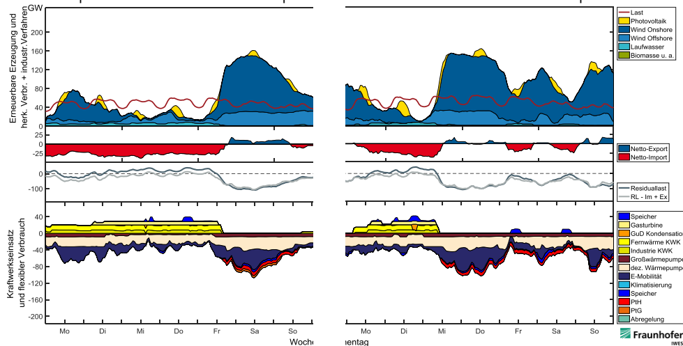
Abbildung 4-26: Zeitpunkt mit höchstem Kraftwerksabruf, Szenariojahr 2050 am Do. 07.01. (links) und Di. 26.01.2010 (rechts) – europäische Versorgungssicherheit
