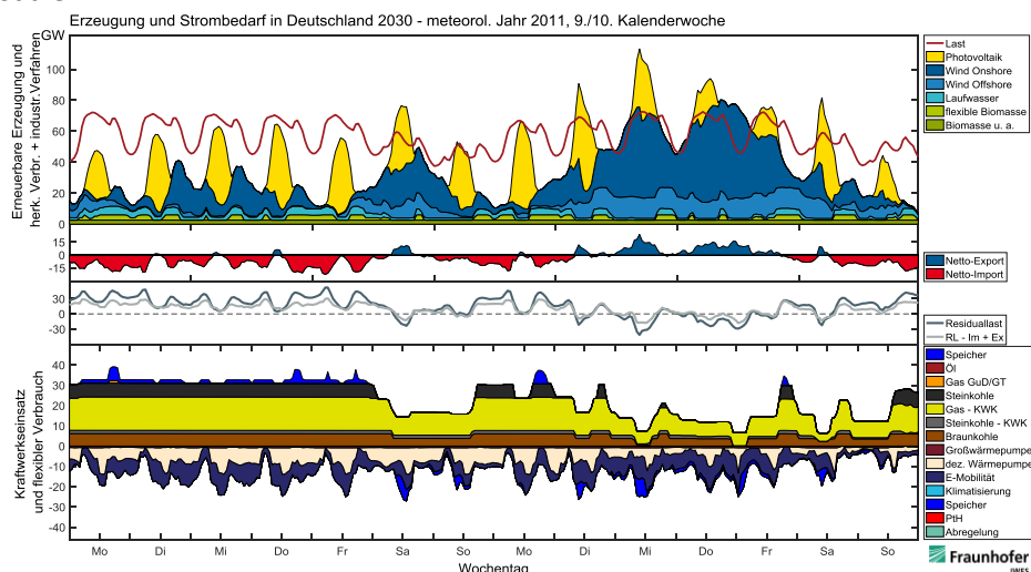
Abbildung 4-29: Verbrauch und Lastdeckung – zwei Beispielwochen Wetterjahr 2011 in Deutschland 2030 – Fokus Import/Export
