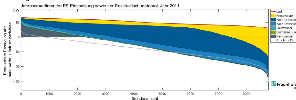
Abbildung 4-14: Jahresdauerlinie EE und unflexibler Verbrauch Wetterjahr 2011 in Deutschland, Szenariojahr 2050
