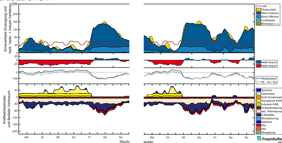
Abbildung 4-27: Zeitpunkt mit höchstem Kraftwerksabruf, Szenariojahr 2050 am Do. 07.01. (links) und Di. 26.01.2010 (rechts) – nationale Versorgungssicherheit und zusätzliche Stromerzeugung für Hybridsysteme
