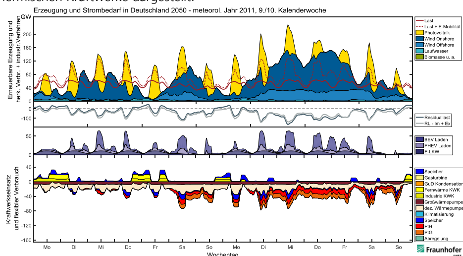
Abbildung 4-11: Verbrauch und Lastdeckung – Zwei Beispielwochen Wetterjahr 2011 in Deutschland, Szenariojahr 2050 – Fokus Elektromobilität
