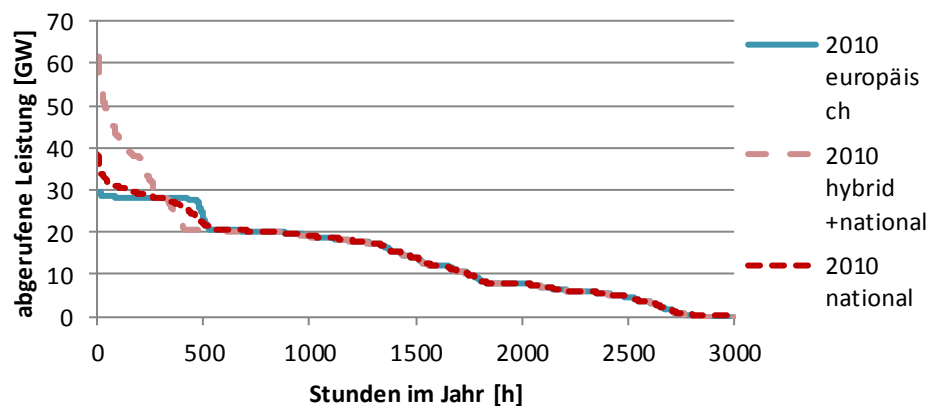
Abbildung 4-25: Jahresdauerlinien der Stromerzeugung aus Gaskraftwerken, Szenariojahr 2050 im Wetterjahr 2010 – Vergleich zwischen europäischer und nationaler Versorgungssicherheit
