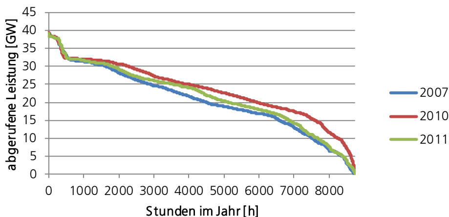
Abbildung 4-30: Jahresdauerlinien der Stromerzeugung aus fossilen thermischen Kraftwerken über drei Wetterjahre, Szenariojahr 2030
