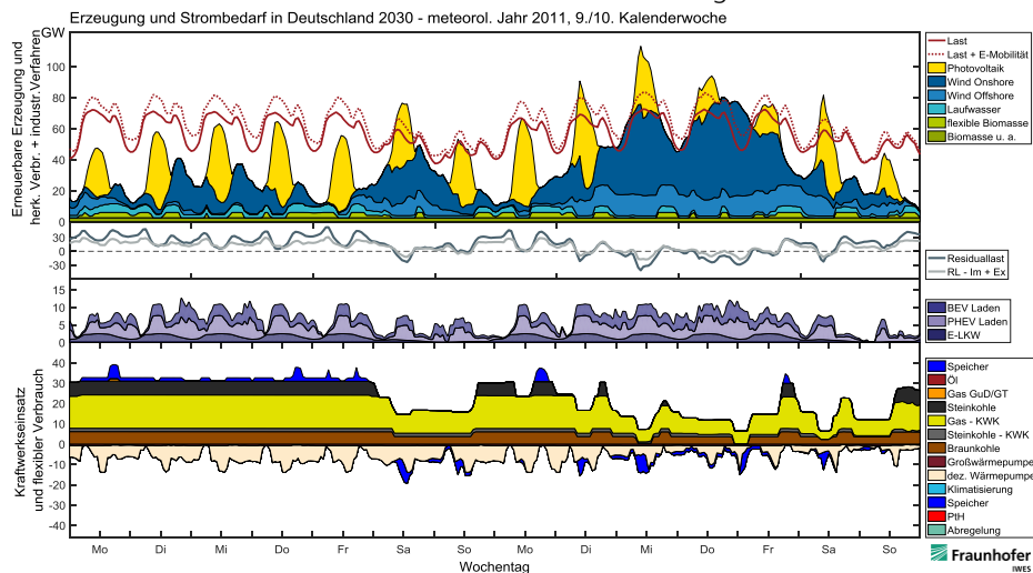
Abbildung 4-28: Verbrauch und Lastdeckung – Zwei Beispielwochen Wetterjahr 2011 in Deutschland 2030 – Fokus Elektromobilität
